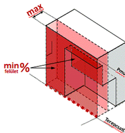
ELTÉRÉSSEL SZABÁLYOZOTT ÉPÍTÉSI VONAL
