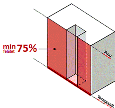
ELTÉRÉSSEL SZABÁLYOZOTT ÉPÍTÉSI VONAL
