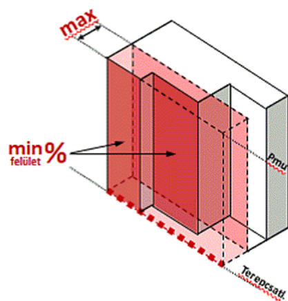
ELTÉRÉSSEL SZABÁLYOZOTT ÉPÍTÉSI VONAL
